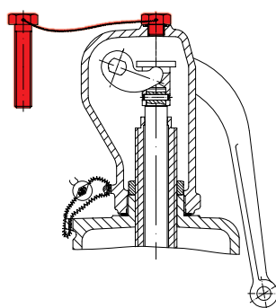
Test gag
