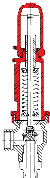
Fig. 25.943 gastight cap
